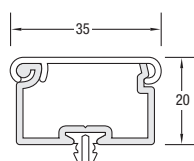
M 1485 Kabelhalteprofil Aluminium, 2480 mm
